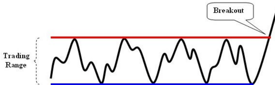
Fig 3.3 - Un esempio di trading range
